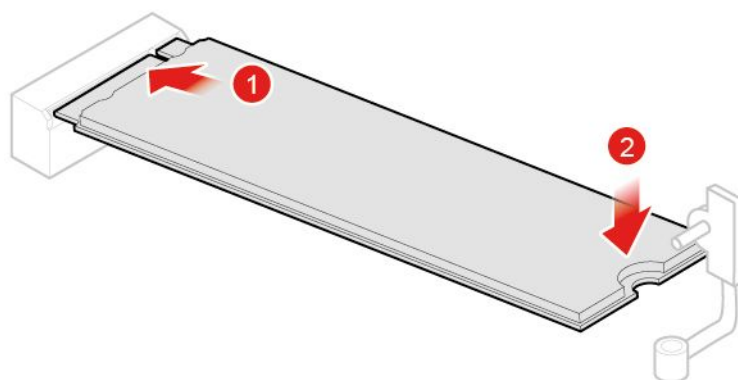
图 92. 安装 M.2 固态硬盘
