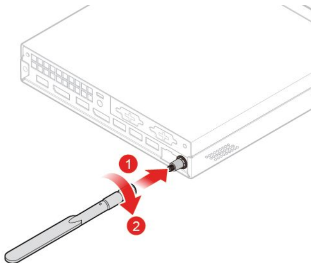
图 80. 安装固定背面 Wi-Fi 天线线缆的天线外盖
